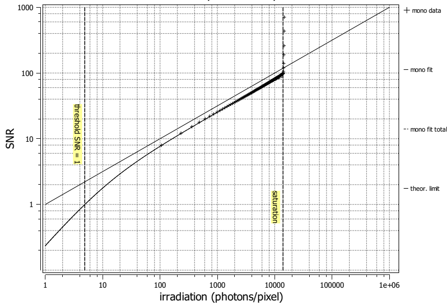
SNR mACC300150, 533 nm, 01.06.2023
