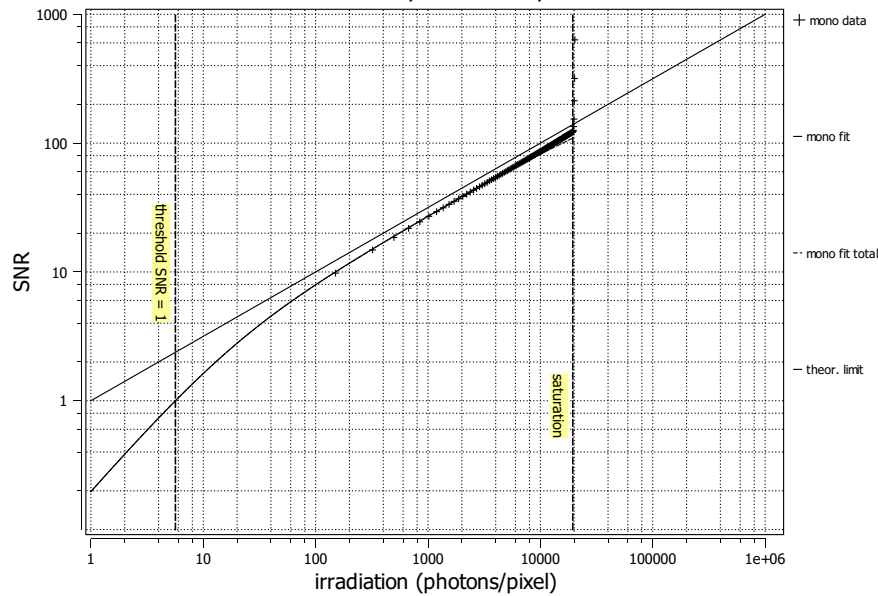
SNR mACC300244, 533 nm, 10.10.2023
