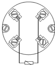
Einzelelement, 2-Leiter
