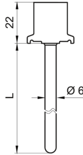
Tri-Clamp Ø 25 (BCID: C01) 3-A
