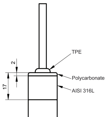
Sortie de câble, 4 conducteurs, 5 m longueur
