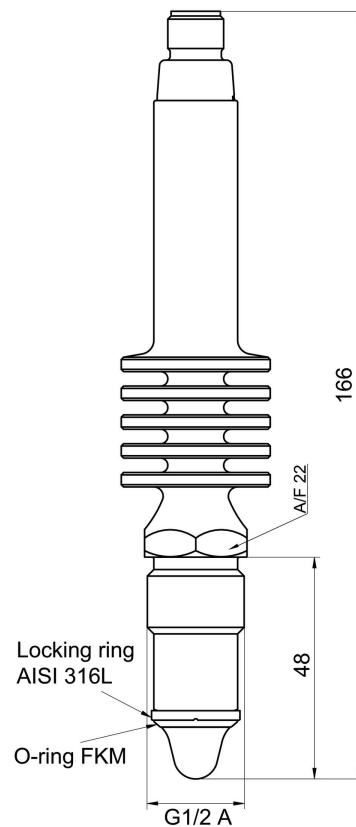
G 1/2 A hygiénique, haute température, avec col de refroidissement (BCID: A03)
