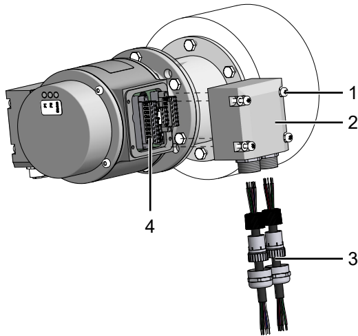
Abb. 10: Anschlusskasten HOG980.M
