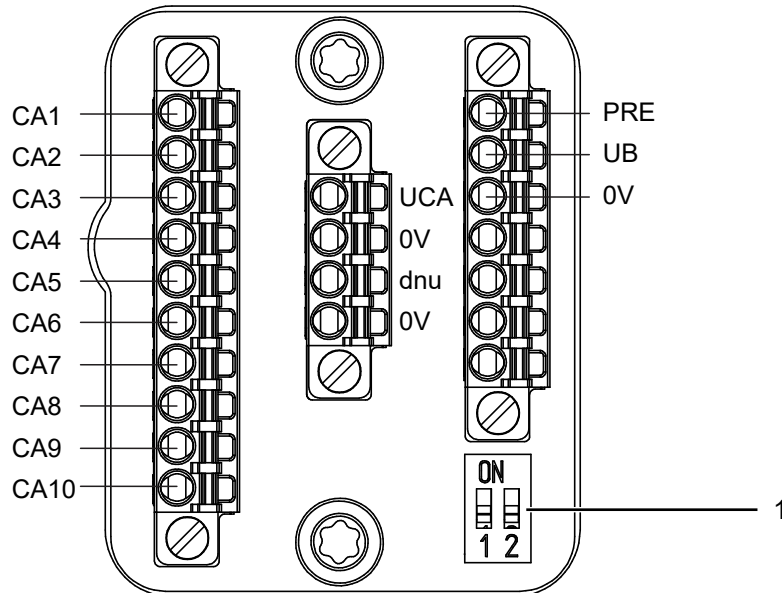
Abb. 11: Anschlussklemmen HOG980.M
