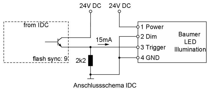
Anschlusschema IDC
