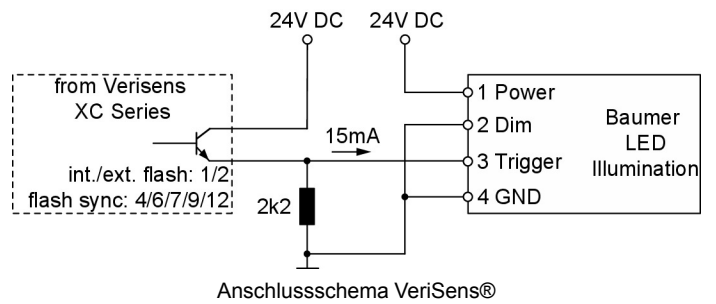
Blitzbetrieb (NPN)
