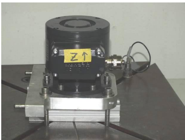
Bild 11 Drehgeber POG 9 auf dem Stoßtisch mit Beschleunigungssensor beim Schocken in der Z-Achse, positive Richtung
