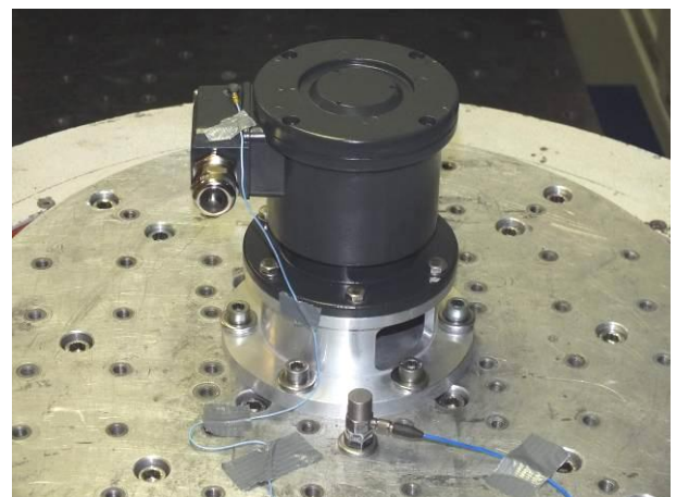
Bild 6 Drehgeber POG 9 auf dem Schwingtisch mit Beschleunigungssensoren beim Schwingen in der Z-Achse
