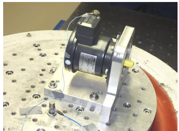
Bild 4 Drehgeber POG 9 auf dem Schwingtisch mit Beschleunigungssensoren beim Schwingen in der Y-Achse
