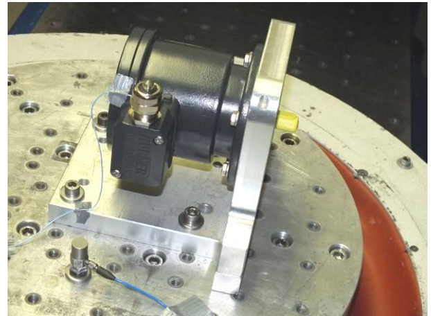
Bild 2 Drehgeber POG 9 auf dem Schwingtisch mit Beschleunigungssensoren beim Schwingen in der X-Achse
